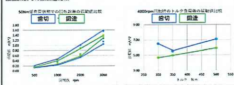
強度試験での振動値比較
